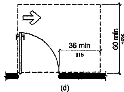
(d) hinge approach, pull side
